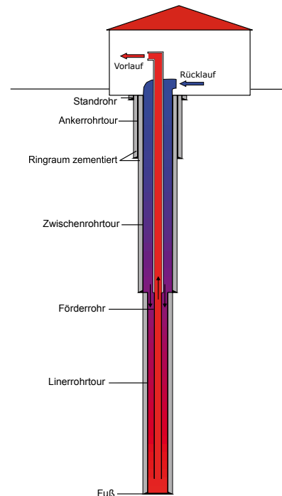
Prinzipiskizze einer geothermischen Erschließung mittels Erdwärmesonde
